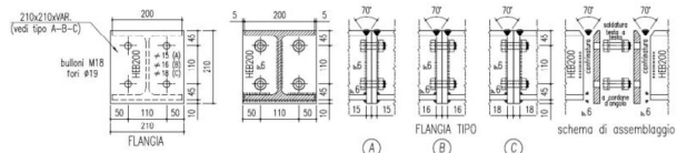
COLLEGAMENTI FLANGIATI SU HEB200 DI ASSEMBLAGGIO DEI PORTALI
